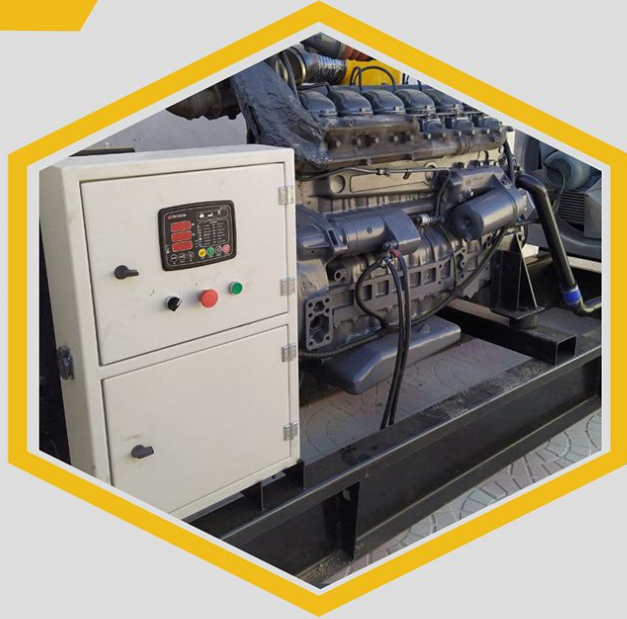
موتور ژنراتور گاز سوز مان
